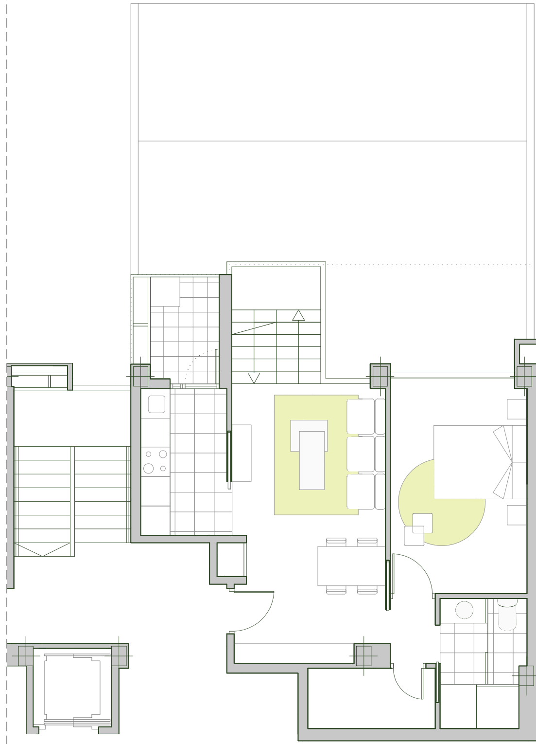
PLANTA ACCESO
